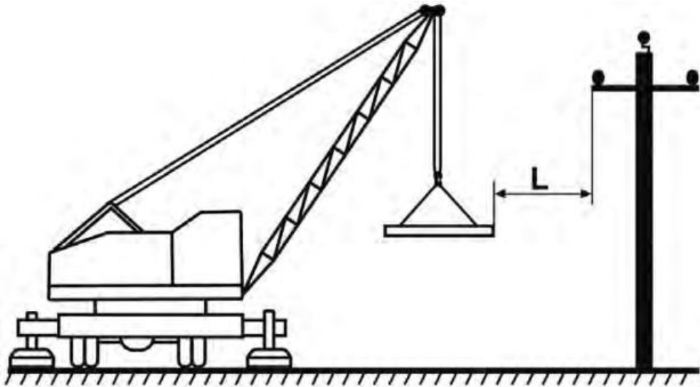
Rys. 4. Maszynę ustawia się w takiej odległości ( L ) od napowietrznej linii elektroenergetycznej, aby zachowane były minimalne odległości mierzone do najdalej wysuniętego punktu urządzenia wraz z ładunkiem.
