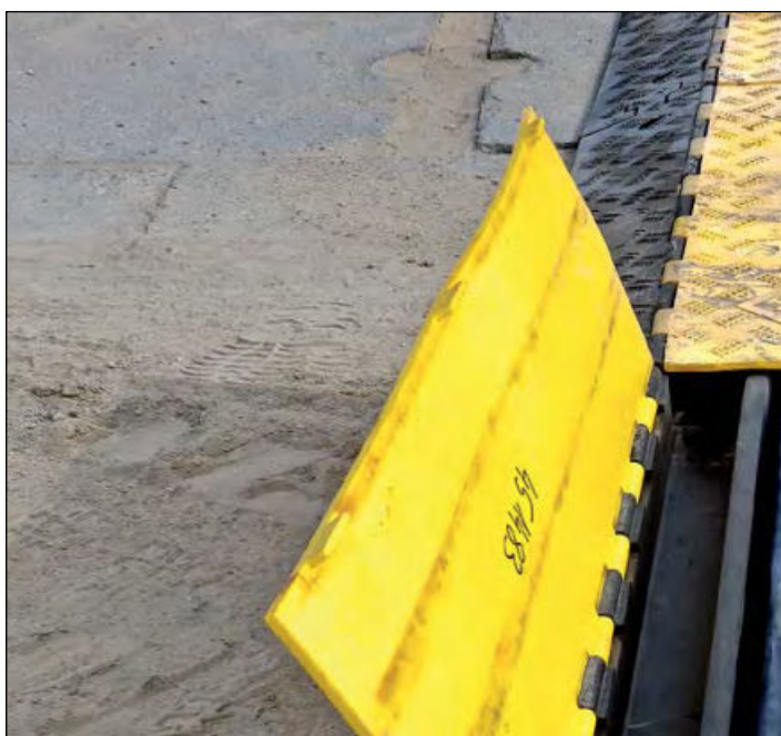
Najazd kablowy gumowy zamykany pokrywą: długość segmentu 90 cm, szerokość 60 cm, wysokość 7,5 cm, dopuszczalny nacisk osi 10 t (5 t na segment).
