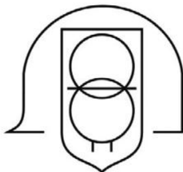
Rys. 6. Oznakowanie transformatora bezpieczeństwa przeznaczonego do stosowania na terenie budowy.
